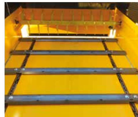
Fond chaînes barrette avec hérisson à dent fixes
